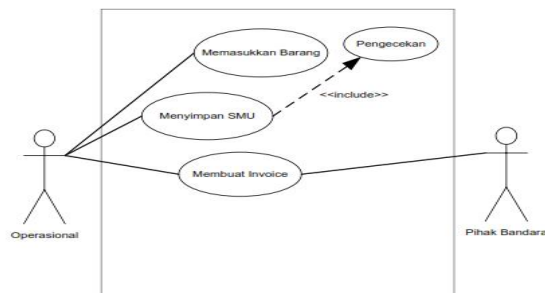
Gambar 11 Use Case Diagram Penyerahan pengiriman barang
