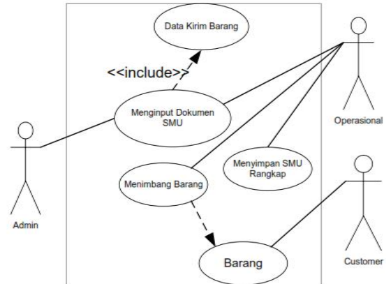
Gambar 10 Use Case Diagram Pengambilan Barang
