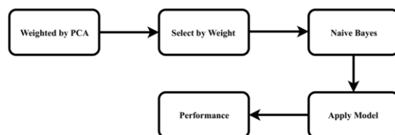
Gambar 4. Langkah Pengujian Naive Bayes dengan Weighted-Principal Component Analysis
