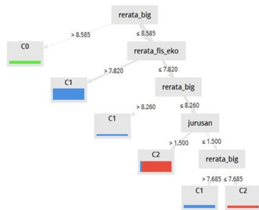
Sumber: (Angraini Yeni, Fauziah Siti, 2020) Gambar3. Pohon keputusan menggunakan algoritma C4.5
