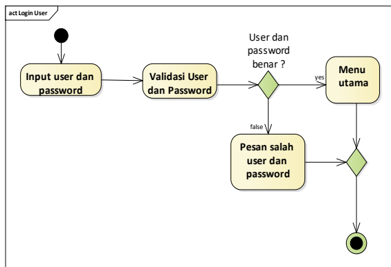
Sumber: (Safitri et al., 2018) Gambar 3. Activity Diagram Sistem Informasi Menu Login
