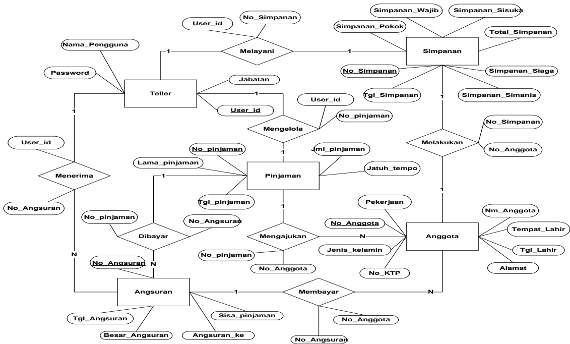
Gambar 6. ER Diagram Sistem Informasi Simpan Pinjam
