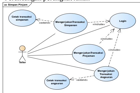
Sumber: (Safitri et al., 2018) Gambar 2. Use Case Diagram Sistem Informasi Simpan Pinjam
