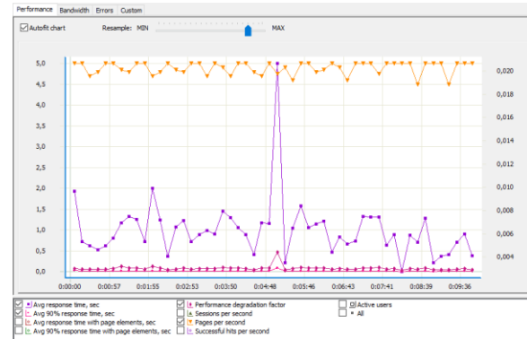
Gambar 11. Hasil Pengujian WAPT
