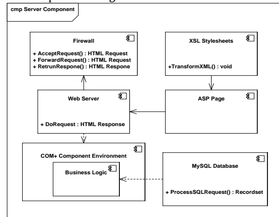
Sumber: (Septiani,2018) Gambar 7. Component Diagram Sistem Manajemen Proyek
