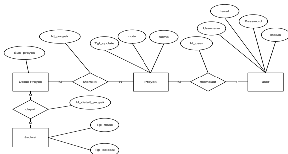
Sumber: (Septiani,2018) Gambar 5. Entity Relationship Diagram (ERD) Sistem Manajemen Proyek
