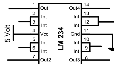
Sumber : Rosano, Yunita & Raharjo (2016) Gambar 3. Rangkaian Penguat LM234
