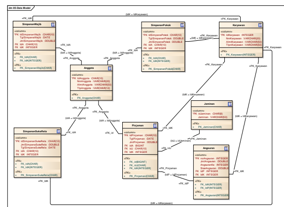
Gambar 8 Data Model Sistem Informasi Koperasi Simpan Pinjam SMK 18 LPPM RI Sidareja
