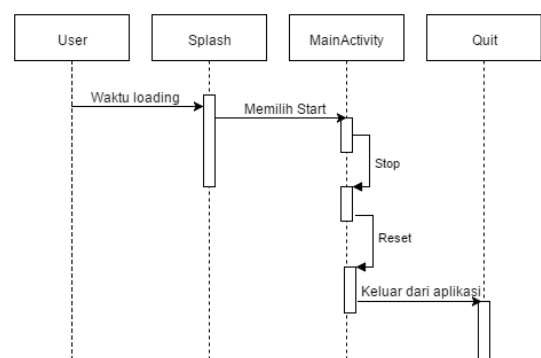
Sumber: hasil analisis(2016) Gambar 4. Sequence diagram menu aplikasi
