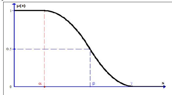
Sumber: (Kusumadewi, S., & Purnomo, 2010) Gambar 7. Grafik Fungsi Keanggotaan Kurva-S Turun
