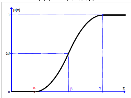
Sumber: (Kusumadewi, S., & Purnomo, 2010) Gambar 6. Grafik Fungsi Keanggotaan Kurva-S Naik
