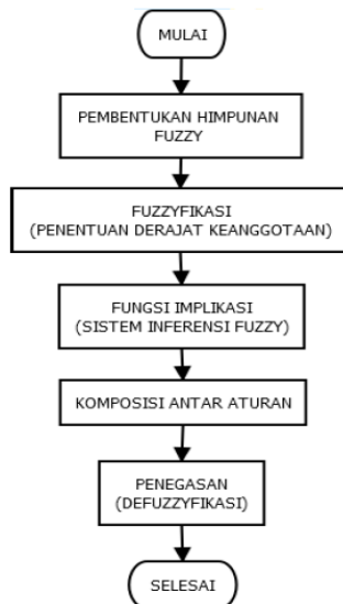
Sumber: (Kusumadewi, S., & Purnomo, 2010) Gambar 1. Flowchart Metode Mamdani
