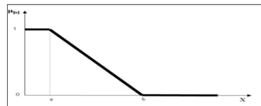
Sumber: (Kusumadewi, S., & Purnomo, 2010) Gambar 3. Grafik Fungsi Keanggotaan Linier Turun
