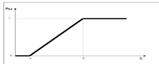
Sumber: (Kusumadewi, S., & Purnomo, 2010) Gambar 2. Grafik Fungsi Keanggotaan Linier Naik
