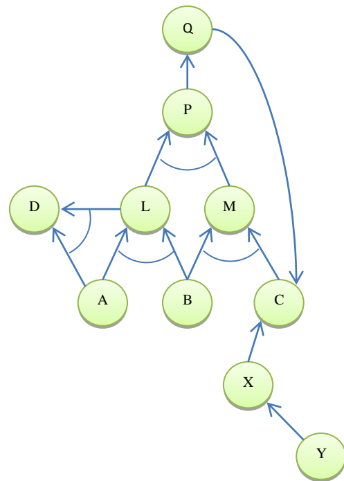
Gambar 3. Pohon Pakar
