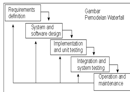
Gambar 1. Pemodelan Waterfall
