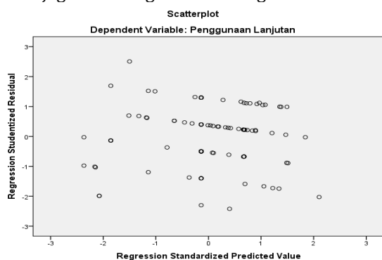
Gambar 2. Grafik Scatterplot
