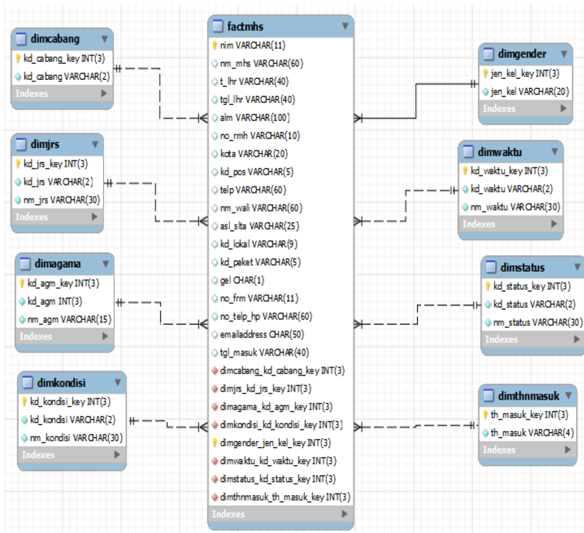
Gambar 6. Star Schema Aplikasi OLAP Data Warehouse Mahasiswa.
