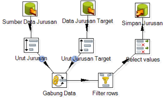
Sumber : Hasil Penelitian (2015) Gambar 11. Staging data dimensi jurusan.
