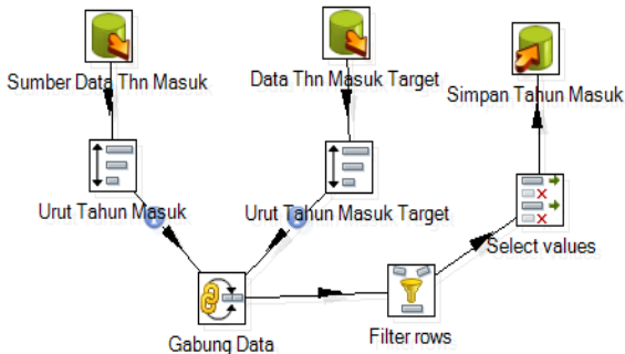
Sumber : Hasil Penelitian (2015) Gambar 14. Staging data dimensi tahun masuk.
