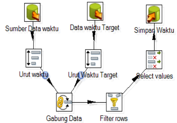
Sumber : Hasil Penelitian (2015) Gambar 15. Staging data dimensi waktu.
