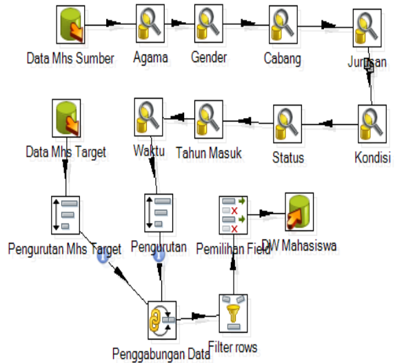
Sumber : Hasil Penelitian (2015) Gambar 16. Staging data fakta mahasiswa.
