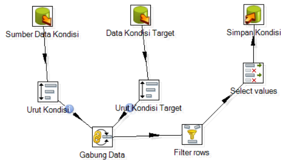
Sumber : Hasil Penelitian (2015) Gambar 12. Staging data dimensi kondisi.
