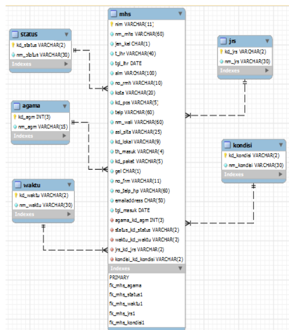
Sumber : Hasil Penelitian (2015) Gambar 3. Skema Database data mahasiswa.
