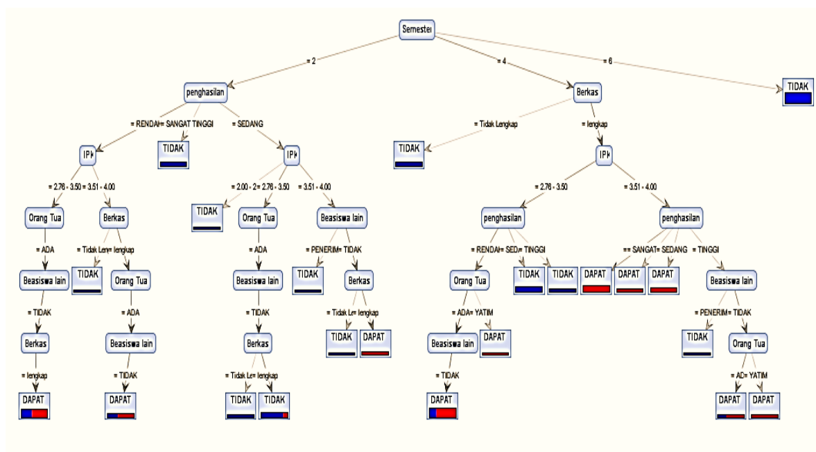
Gambar 2. Decision Tree Klasifikasi mahasiswa dengan C4.5
