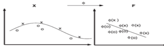
Gambar 1. Kernel map mengubah problem yang tidak linier menjadi linier dalam space baru
