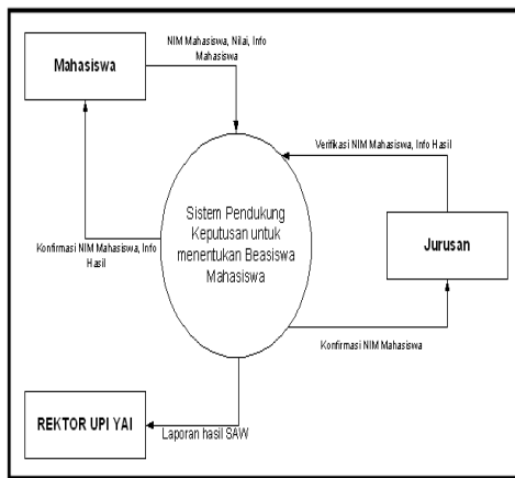
Gambar 2. Diagram Konteks
