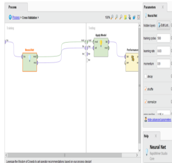
Sumber : (Rahayu et al., 2019) Gambar 7. Proses Insert Model NN Yang Akan DiTraining
