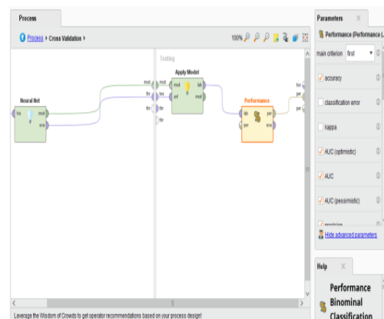
Sumber : (Rahayu et al., 2019) Gambar 8. Proses Testing Dengan Cara Insert Apply Model dan Performance
