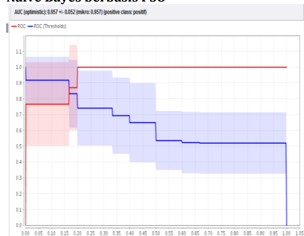
Gambar 2 Kurva ROC Naive Bayes dan PSO
