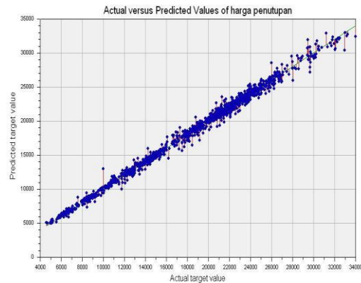
Gambar 4 Nilai yang diprediksi terhadap nilai yang sebenarnya dalam hal harga pada MLP (6-3-1)
