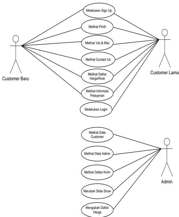
Sumber: (Hasil Penelitian, 2015) Gambar 6 Use Case Diagram Penyampaian Informasi Pengiriman Barang
