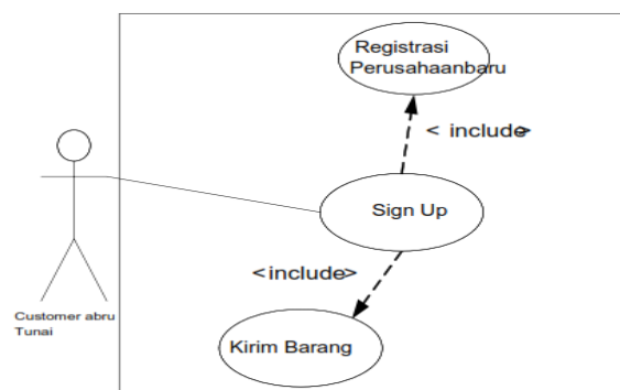
Sumber: (Hasil Penelitian, 2015) Gambar 8 Use Case Diagram Registrasi Customer Baru Pembayaran Tunai
