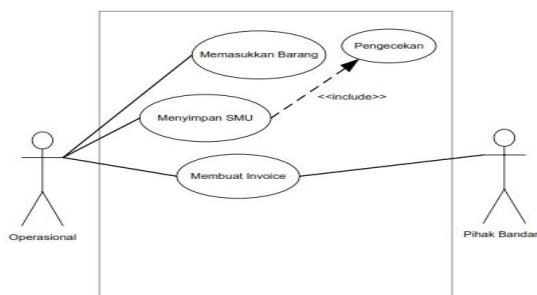
Gambar 11 Use Case Diagram Penyerahan pengiriman barang
