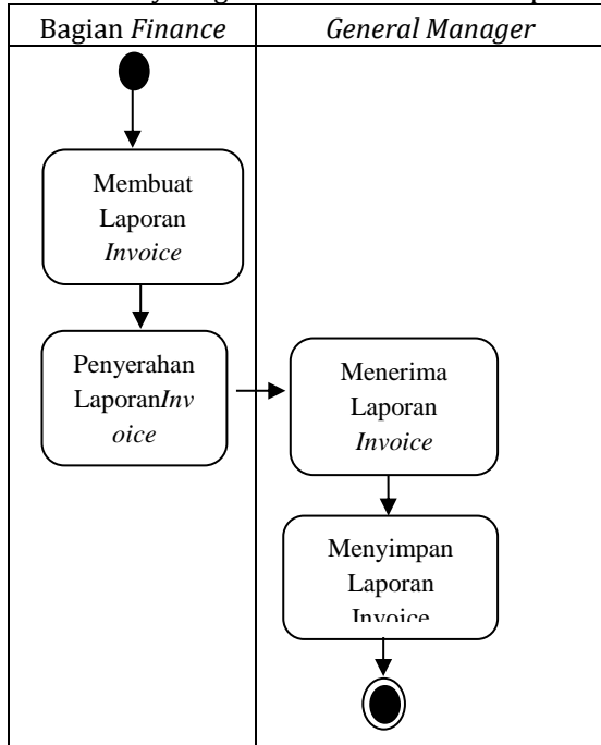
Sumber: (Hasil Penelitian, 2015) Gambar 4 Activity Diagram Proses Pembuatan laporan
