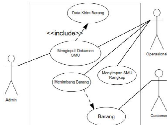
Gambar 10 Use Case Diagram Pengambilan Barang
