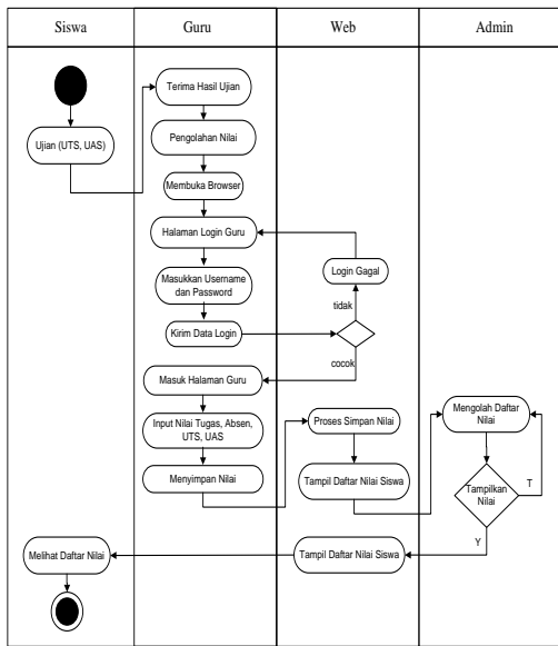
Sumber : Fitriani (2018) Gambar 7. Activity Diagram Informasi Daftar Nilai Siswa
