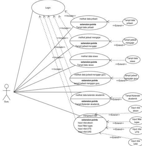
Sumber : Fitriani (2018) Gambar 3. Use Case Diagram Akademik Sekolah Online Halaman Guru
