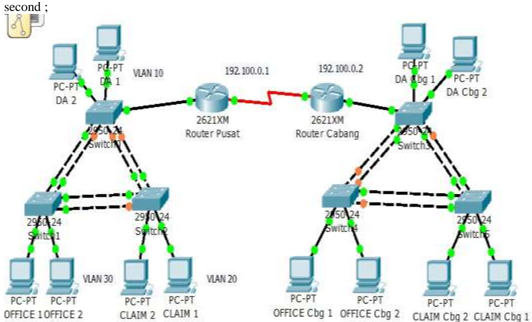
Gambar 5. Jaringan Akhir
