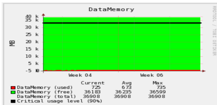
Gambar 9. Memory Usage setelah mekanisme Load-balancing Clusters
