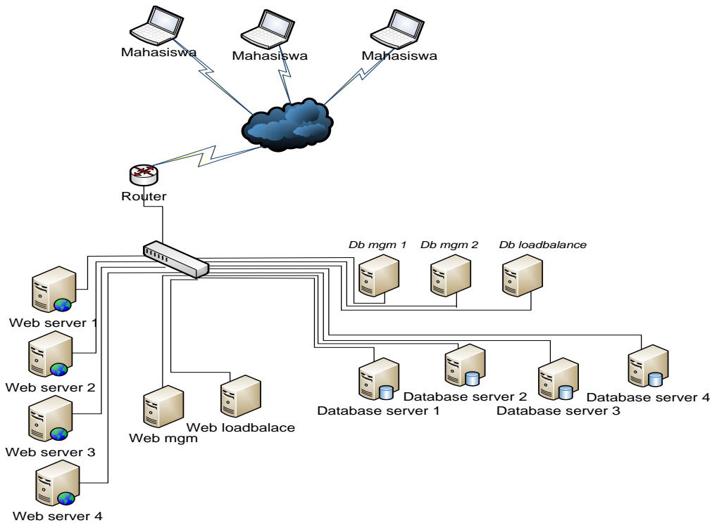
Gambar 3. Topologi Jaringan loadbalance clusters pada database server
